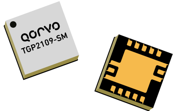
QFN 4x4 mm 16L
